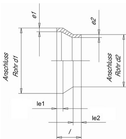
Муфта редукционная PP-H Simona 110x90 SDR17.6 PN10
