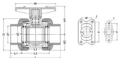
Шаровой кран IVKD ПВДФ с муфтовыми окончаниями d32 (DN25)
