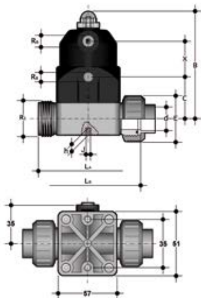
Компактный мембранный клапан СМ ПВДФ с разборными муфтовыми окончаниями d20 (DN15)
