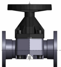
Мембранный клапан VMOV PBX с фланцевыми окончаниями, PTFE, FIP d90 (DN80)
