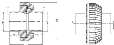
Муфта разборная ПВДФ d90 PN 16
