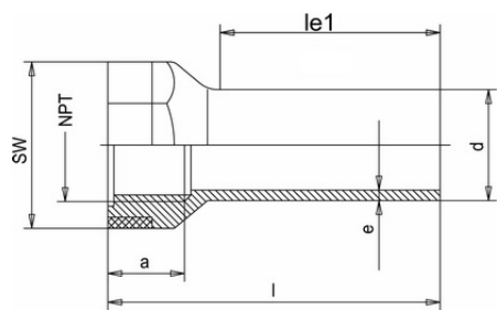
Адаптер переходной с внутренней резьбой ПВДФ (Simona) 20x1/2" SDR21 PN16
