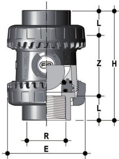
Шаровой обратный клапан SXEJV ПВХ; с резьбовыми окончаниям, FKM, FIP R1¼" (DN32)
