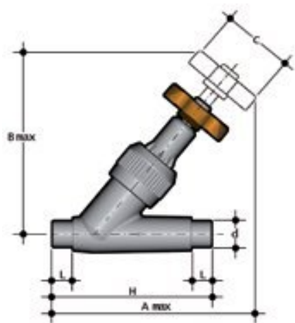
Угловой вентиль VVDV ПВХ с втулочными окончаниями, EPDM, FIP d32 (DN25)
