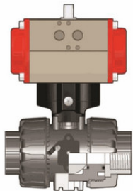
Шаровой кран VKD с пневмоприводом НЗ с резьбовыми окончаниями (уплотнение EPDM) PP-H R3/4" (DN20)
