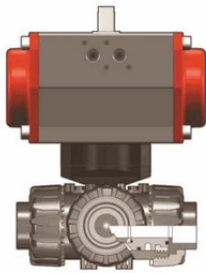
3-х ходовой шаровой кран ТКД ПБХ с пневмоприводом, Т-шар, FIP d50 (DN40)
