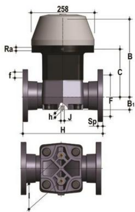
Мембранный клапан VM с пневмоприводом НЗ, PN10 с фланцевыми окончаниями (уплотнение FKM/мембрана FKM) PP-H d90 (DN80)
