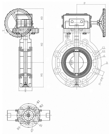
Затвор дисковый в корпусе FRPP (диск - ХПВХ) с редуктором промышленного применения EPDM IPS d225 (DN200)
