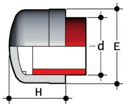
Заглушка для раструбной сварки PP-H FIP d20 PN10
