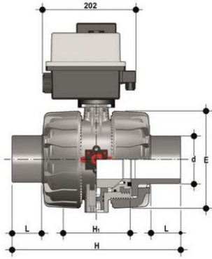
Шаровой кран VKD ПВДФ с эл.приводом 90-240V, втулочные окончания d75 (DN65)
