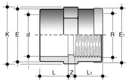
Муфта переходная с ВР и усиливающим кольцом ПВХ FIP 20x1/2
