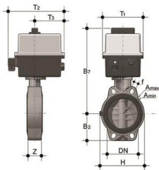
Дисковый затвор общего применения FE ПВХ с эл.приводом 24V AC/DC, EPDM, FIP d63 (DN50)
