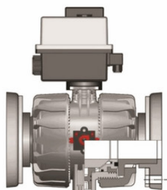
Шаровой кран промышленного применения VKD PBX с электроприводом, FIP d75 (DN65)
