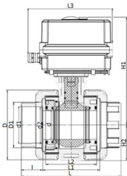
Шаровой кран IVKD ХПВХ с эл.приводом 220V AC, муфтовые окончания d110 (DN100)
