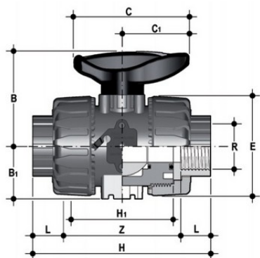
Шаровой кран ПВХ промышленного применения VKD с резьбовыми окончаниями, FKM, FIP R4'' (DN100)
