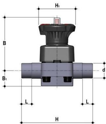
Мембранный клапан DK ХПВХ с втулочными окончаниями d20 (DN15)
