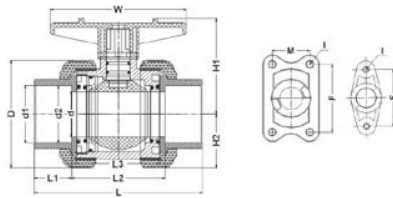
Кран шаровой ПВХ муфтовый общего применения IPS d50
