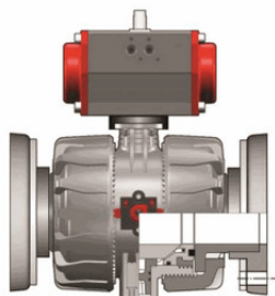
Шаровой кран промышленного применения VKD PBX с пневмоприводом, FIP d90 (DN80)
