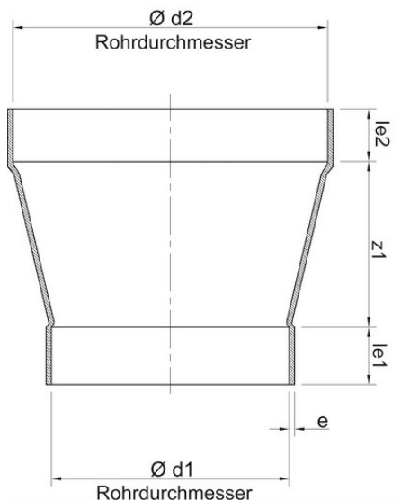
Муфта переходная PPs 560x450
