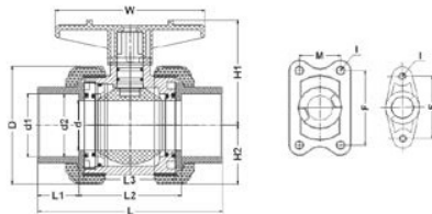
Кран шаровой ПВХ муфтовый общего применения IPS d32
