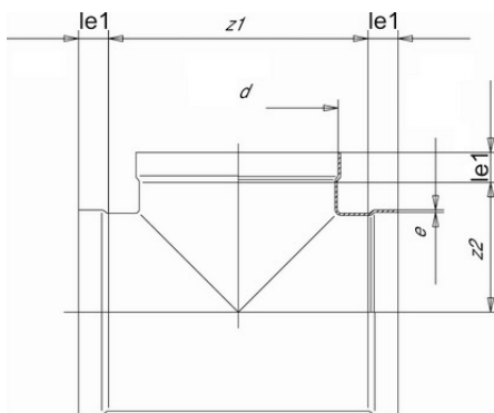
Тройник равнопроходной PPs d500
