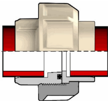
Муфта разборная ПВДФ d63 SDR21 PN16
