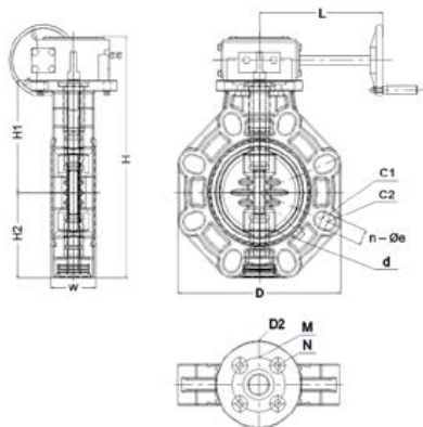
Затвор дисковый с редуктором PP-H IPS (Model A) 10"(DN250)
