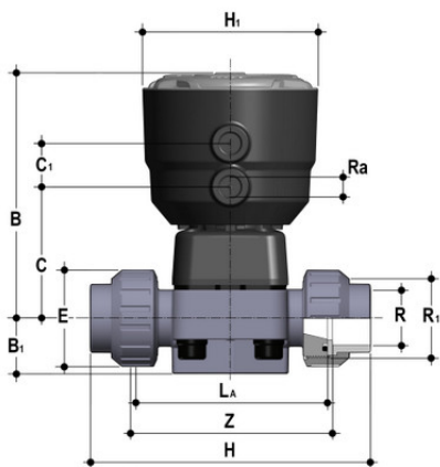
Мембранный клапан DK с пневмоприводом НЗ, PN6 с муфтовыми окончаниями (уплотнение EPDM/мембрана EPDM) PP-H d20 (DN15)
