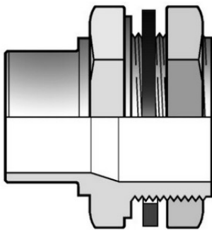
Соединитель с цистерной, LIV ПВХ FIP 25x1
