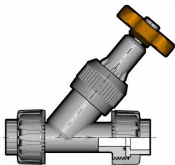
Угловой вентиль VVUIV PBX с разборными муфтовыми окончаниями, EPDM, FIP d50 (DN40)
