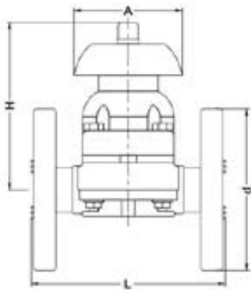
Мембранный клапан с фланцевыми окончаниями PP-H IPS d20 (DN15)
