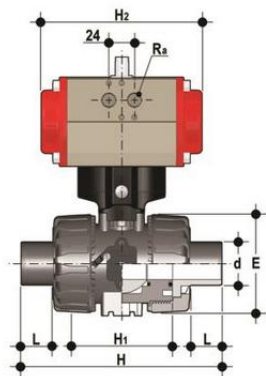
Шаровой кран VKD с пневмоприводом НО с удлинёнными патрубками из ПП (уплотнение FKM) PP-H d63 (DN50)
