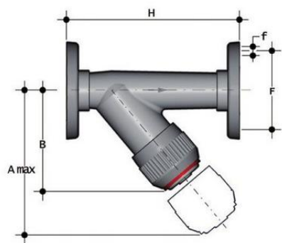
Грязевый фильтр RVOT ПВХ с фланцевыми окончаниями, EPDM, FIP d50 (DN40)
