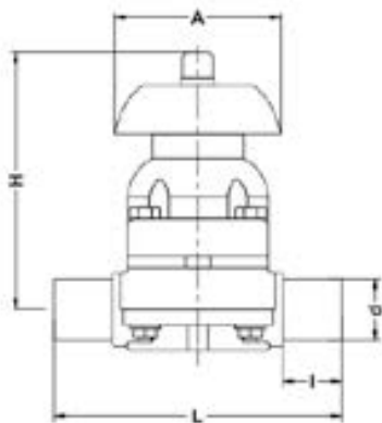
Мембранный клапан с втулочными окончаниями ХПВХ IPS d75 (DN65)
