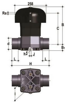
Мембранный клапан VM ПВХ с пневмоприводом НЗ, втулочные окончания, FKM, FIP d90 (DN80)
