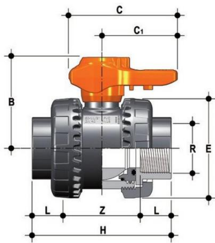
Шаровой кран общего применения VXE ХПВХ с резьбовыми окончаниями R1½" (DN32)
