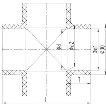
Крестовина клеевая ПВХ IPS d110
