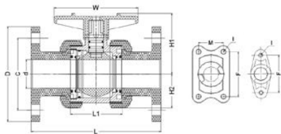
Кран шаровой промышленного применения с фланцевыми окончаниями PP-H IPS d90
