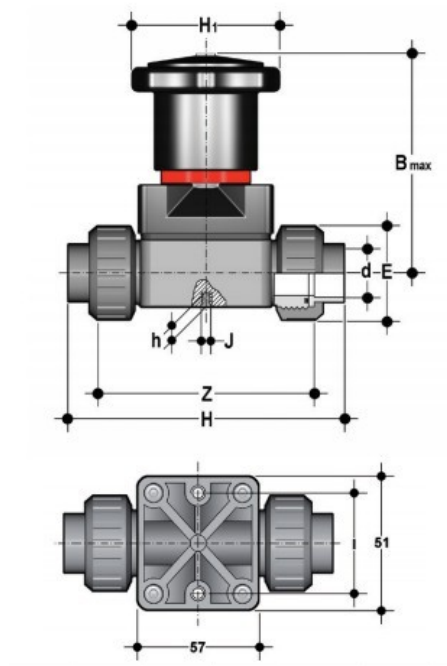
Компактный мембранный клапан CMFV ПВХ с резьбовыми окончаниями, PTFE, FIP d15 (DN15)
