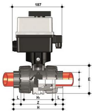
Шаровой кран VKD с эл.приводом 90-240V, муфтовые окончания (уплотнение EPDM) PP-H d25 (DN20)
