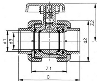
Шаровой кран ПВХ промышленного применения с муфтовыми окончаниями, EPDM, VDL d110 (DN100)
