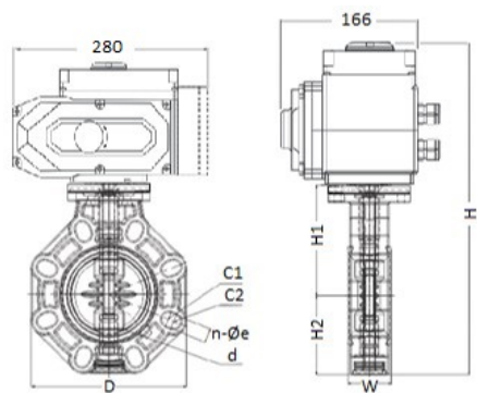
Дисковый затвор IFK ПВХ с электрическим приводом 24V DC, EPDM, IPS d160 (DN150)
