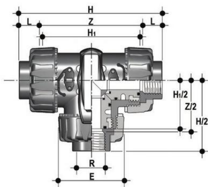
3-х ходовой шаровой кран ТКД ХПВХ с резьбовыми окончаниями, L-шар R3/4" (DN20)
