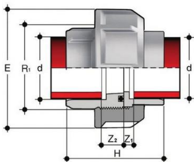
Муфта разборная для раструбной сварки PP-H FIP d63 PN10
