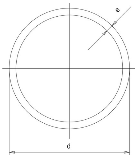
Труба ПВДФ (Simona) d140 SDR33 PN10
