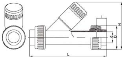
Фильтр сетчатый (грязевой) PP-H IPS d63 (DN50)
