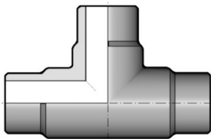
Тройник равнопроходной для стыковой сварки PP-H FIP (PN10) d315 SDR11 PN10
