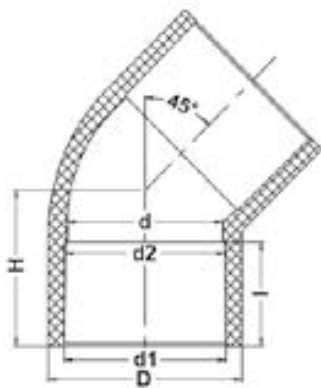
Отвод 45° ХПВХ IPS (Model A) d20 PN16
