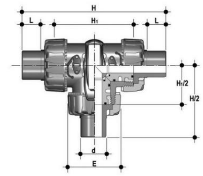
3-х ходовой шаровой кран ТКД с втулочными окончаниями L-шар (уплотнение EPDM) PP-H d32 (DN25)
