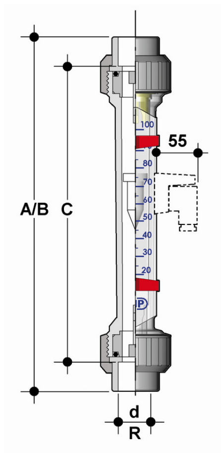
FC ротаметр для воды; корпус: трогамид; поплавок с магнитом d32
